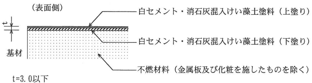
図1 断面図
