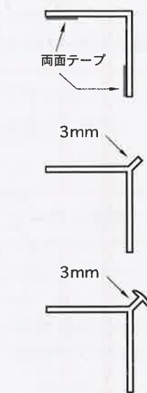
出隅用コーナー定木の種類
