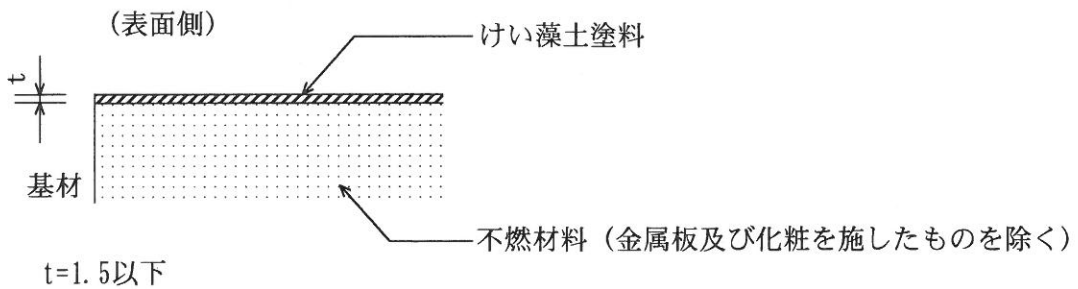
図1 断面図
