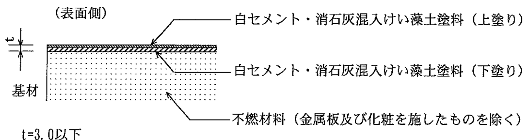
図1 断面図
